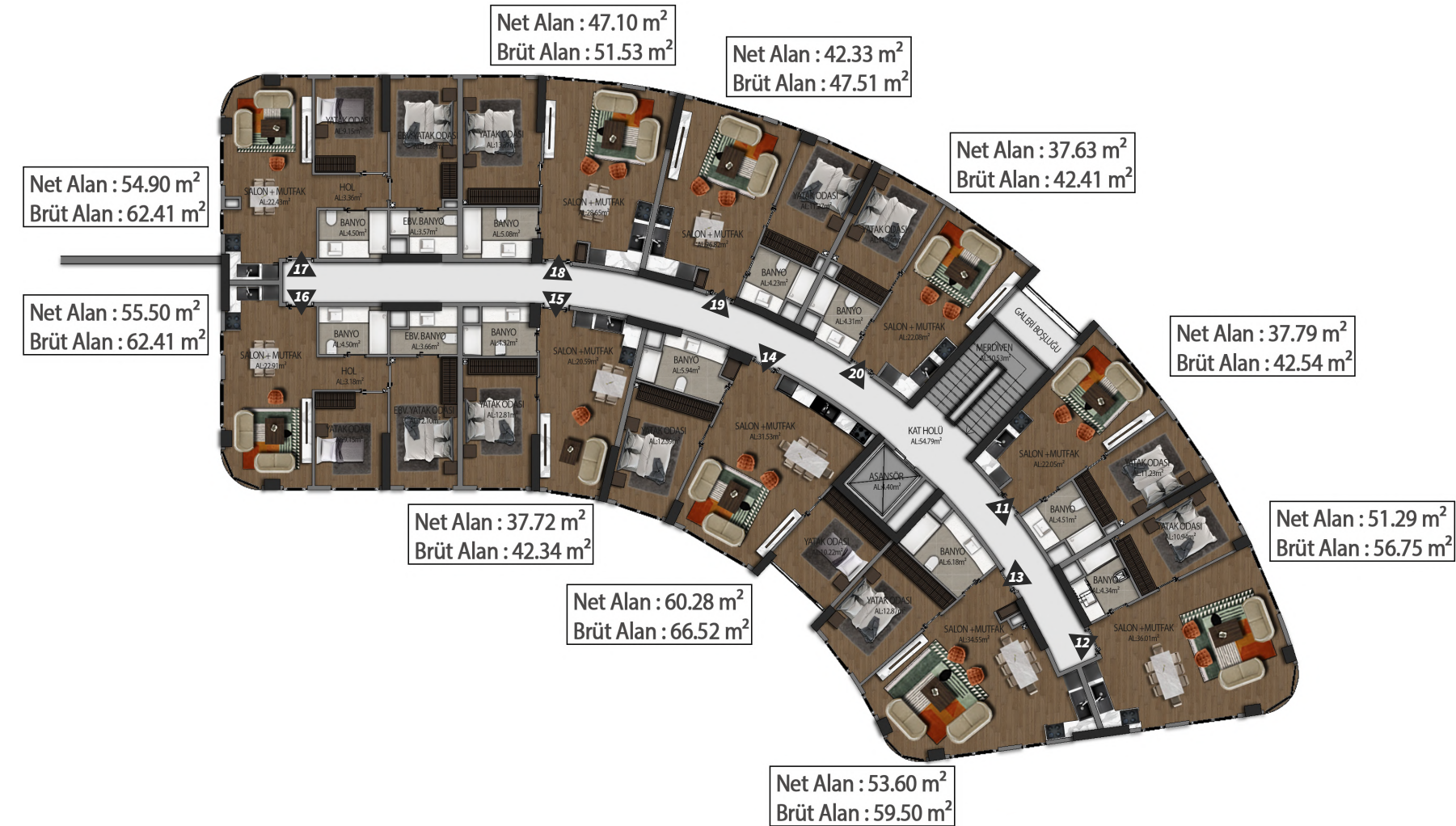
2. Kat Planı
