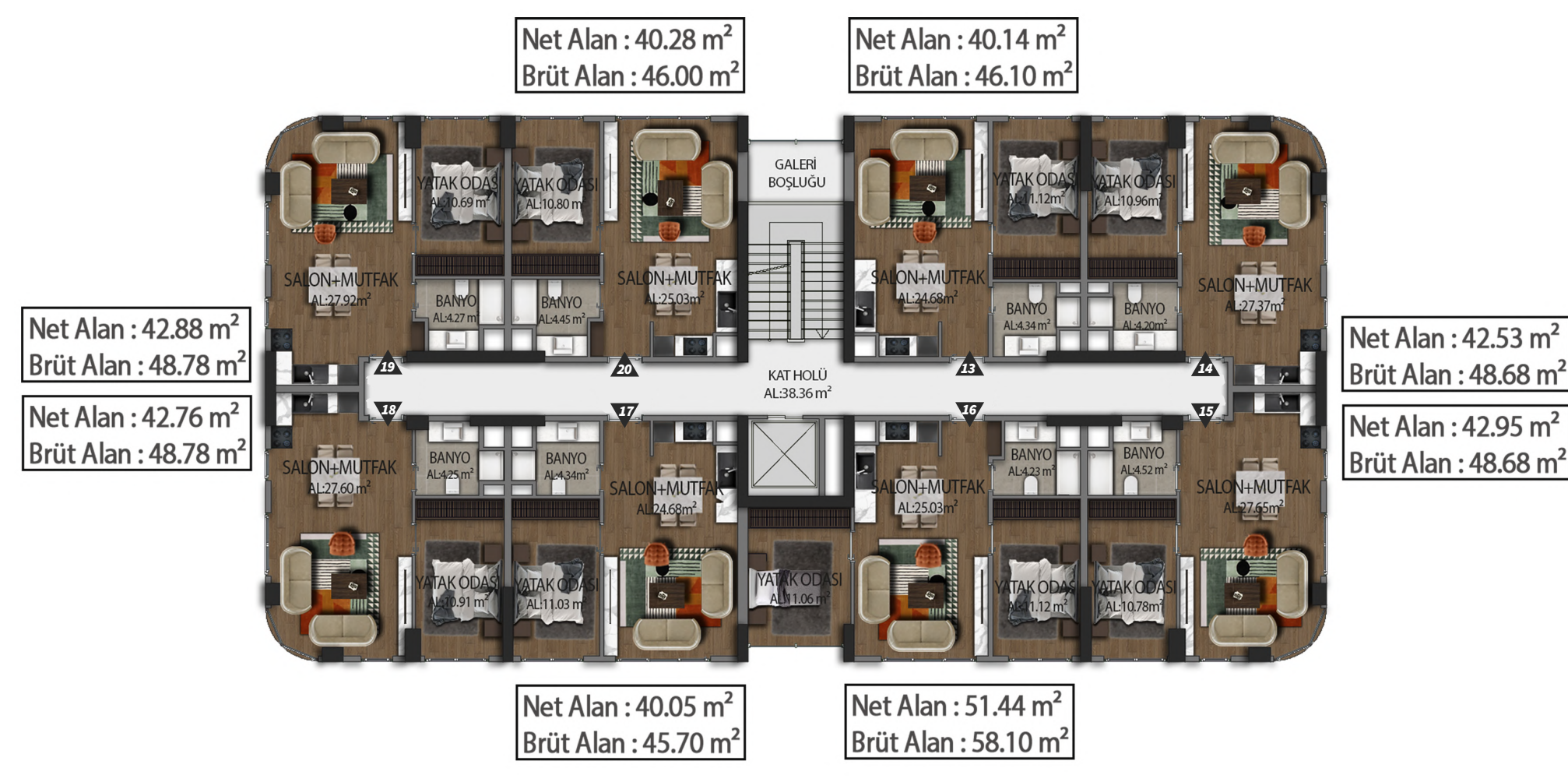
2. Kat Planı
